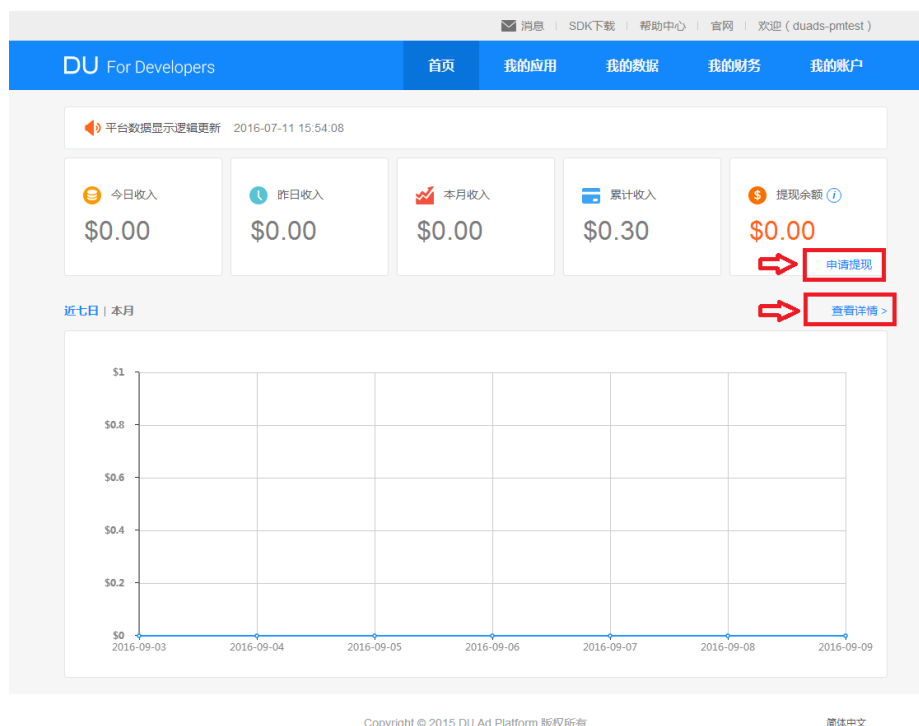
图 3-2-2 平台首页
