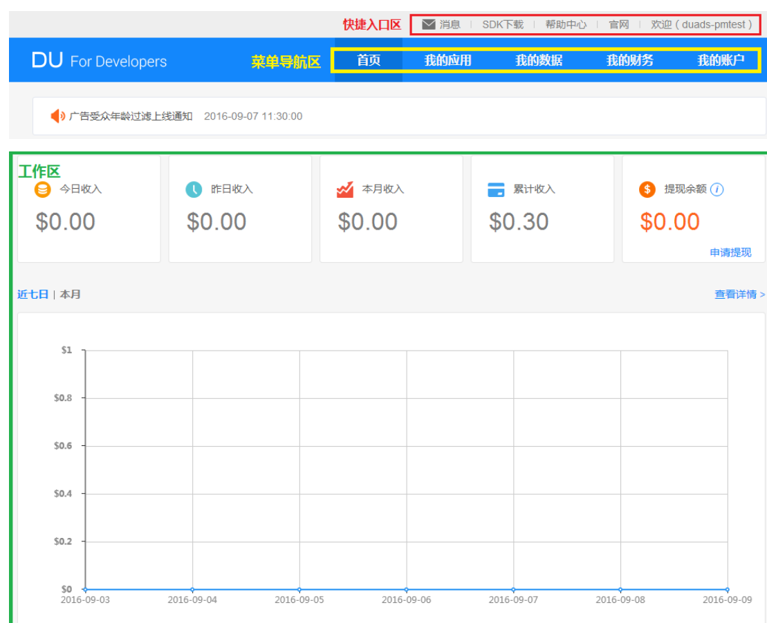
图 2-3-1 平台框架
