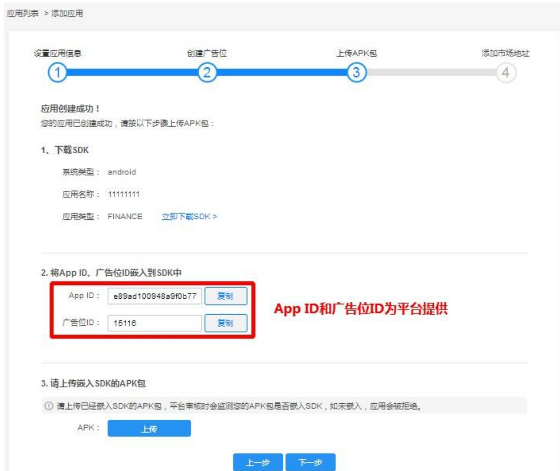
图 3-3-6 上传应用
